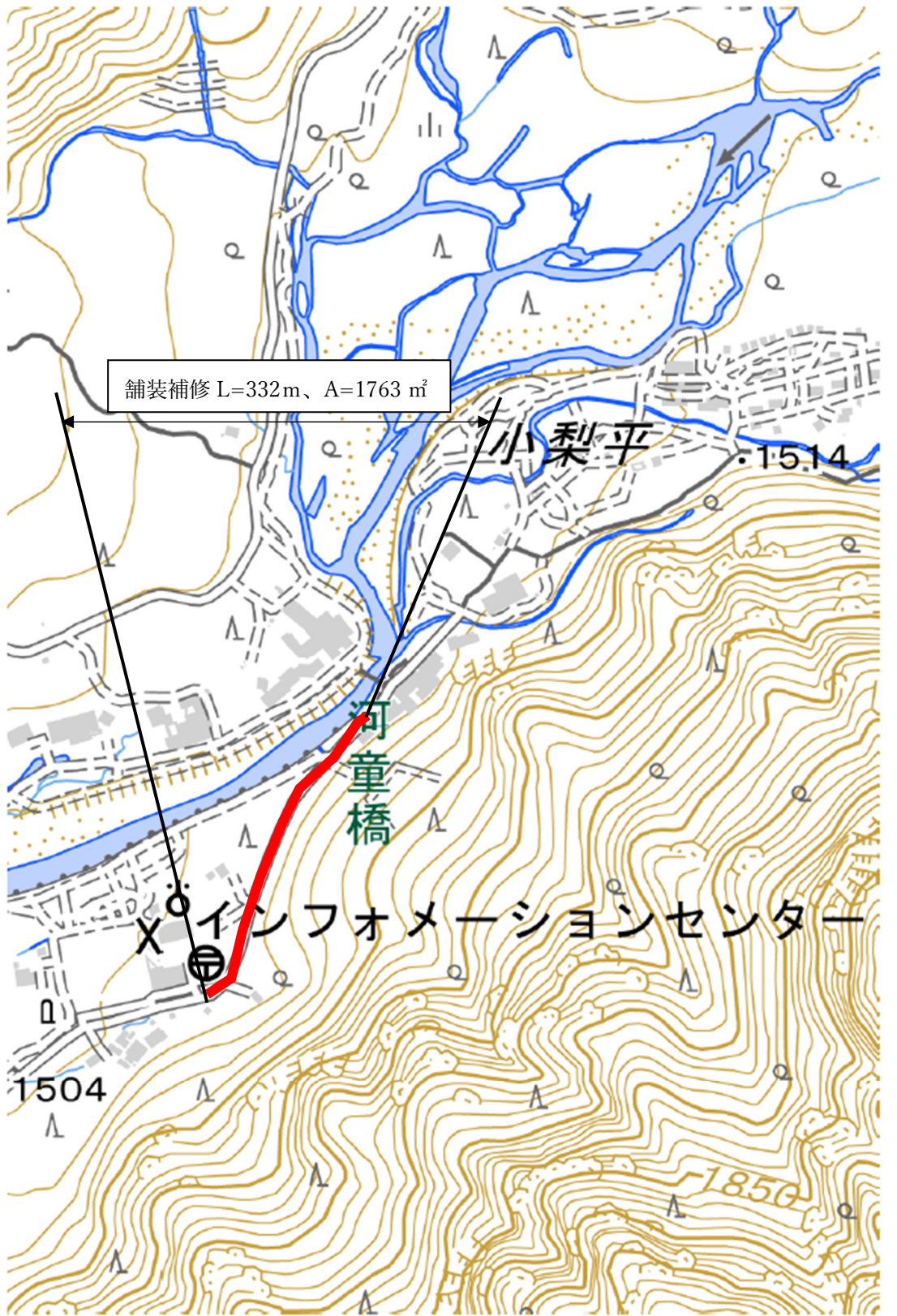
位置図 (1:5000)
