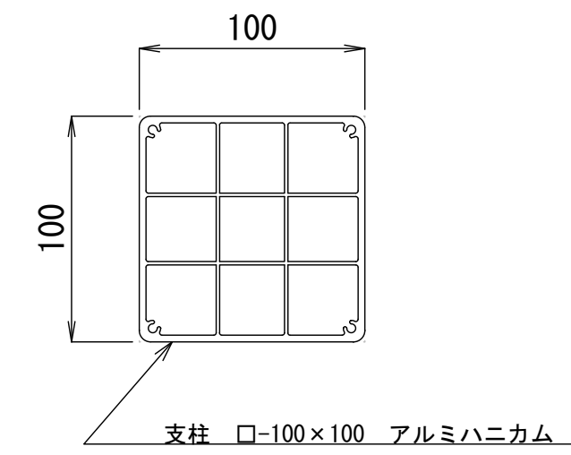
支柱断面図 S=1/3(A1) 、 S=1/6(A3)
