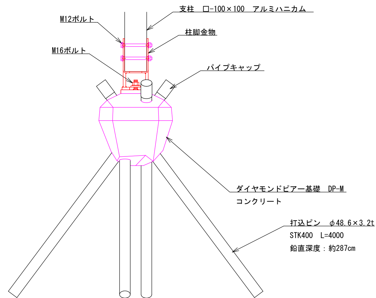
基礎詳細図 ～ダイヤモンドピア基礎 DP-M～
