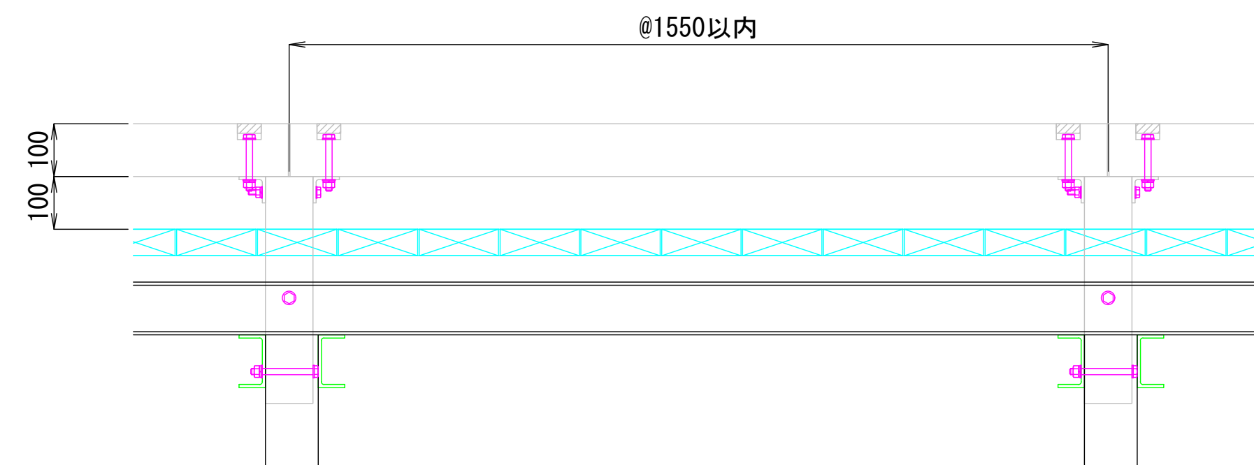
地 覆 詳 細 図
