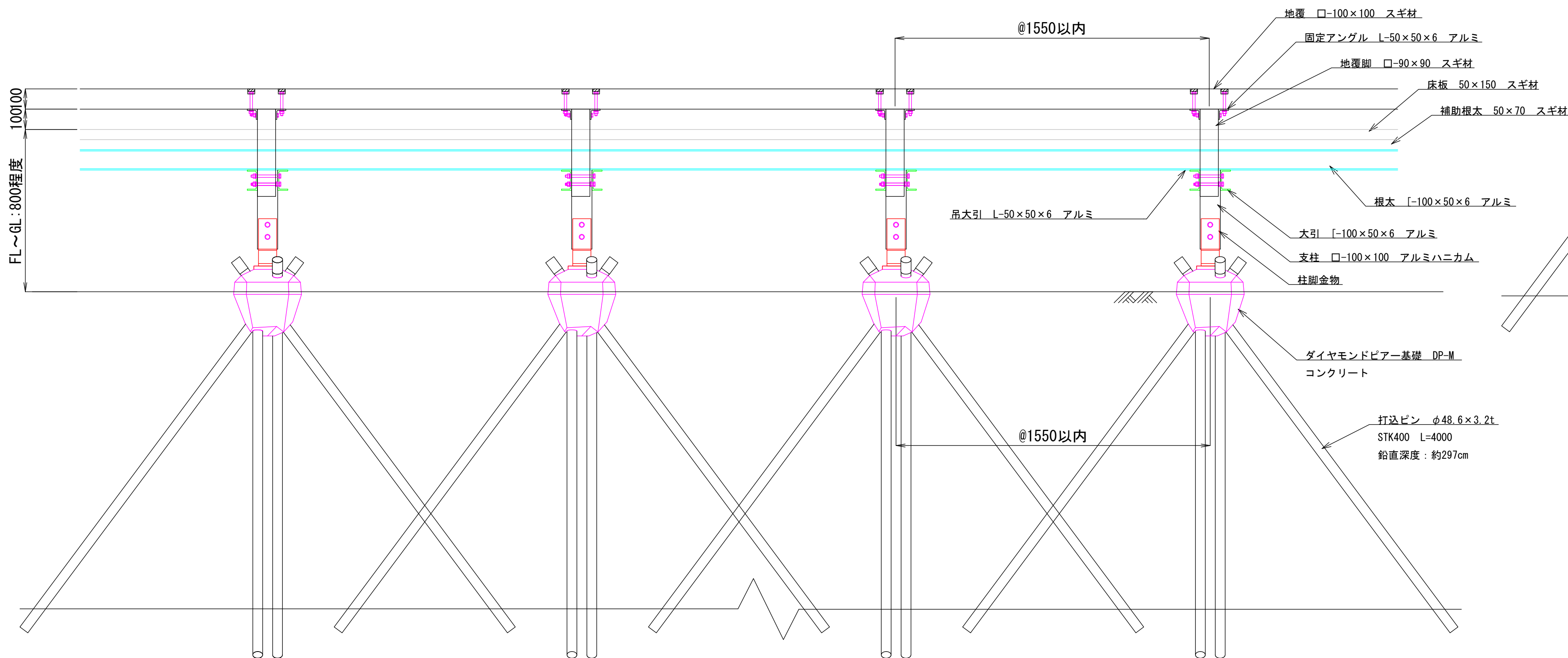
立面図 S=1/15
