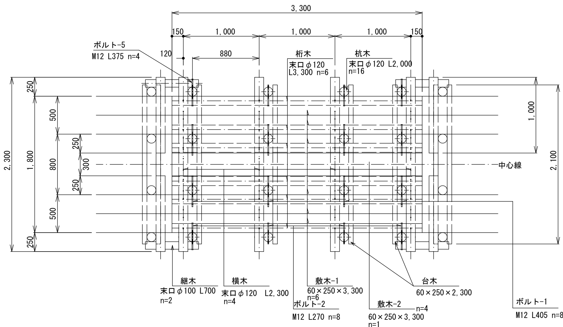
平面図
