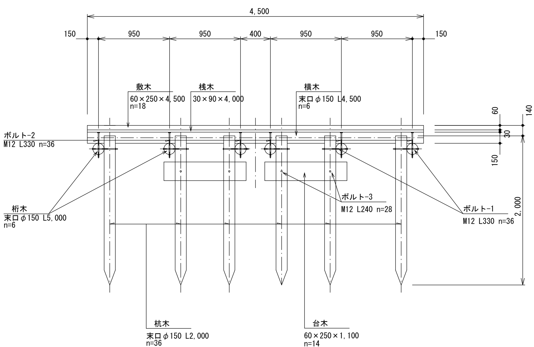
断面図 C--C
