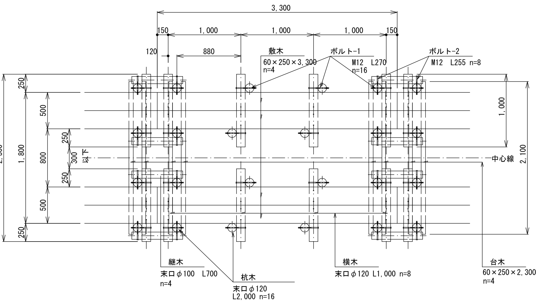
平面図
