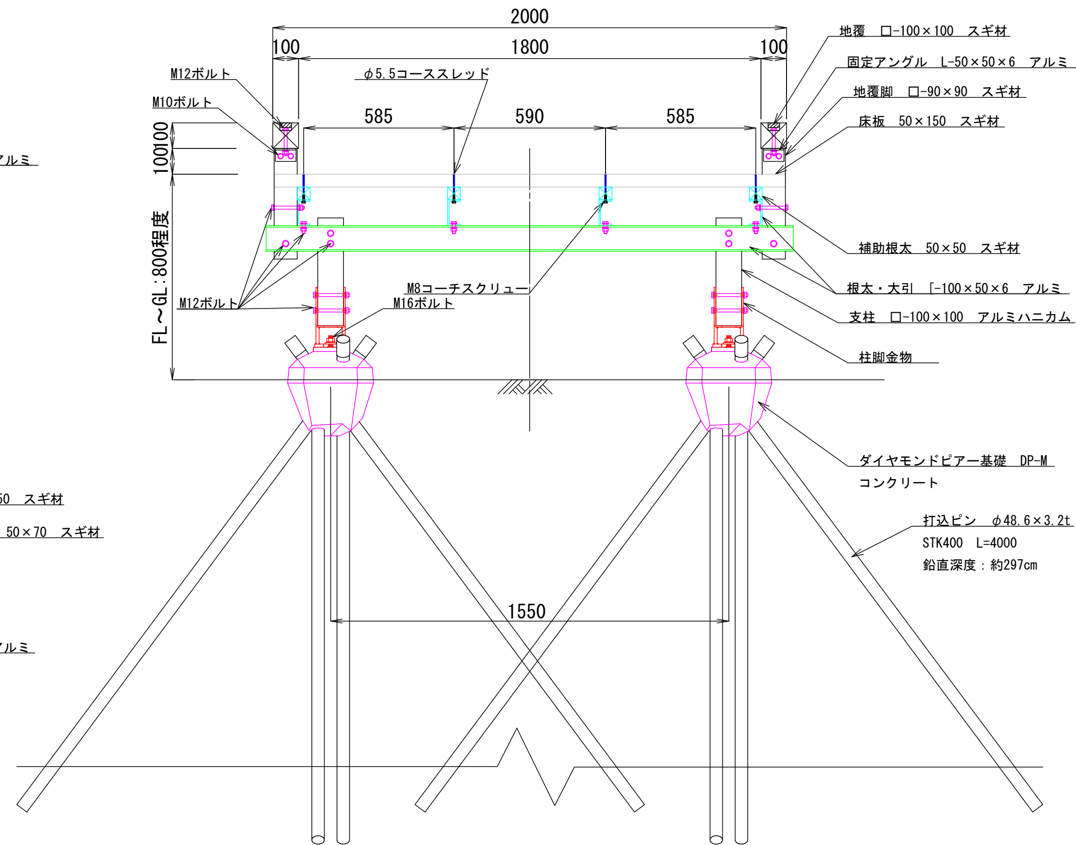
断面図 S=1/15
