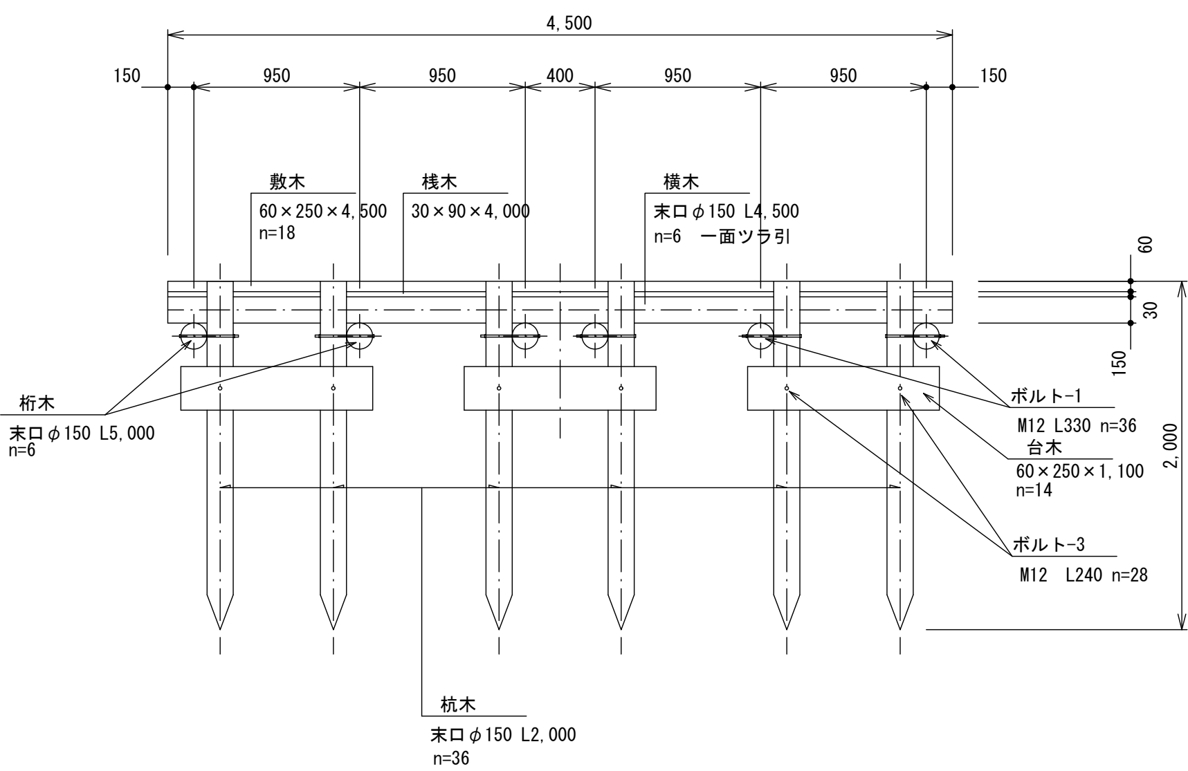
断面図 C--C
