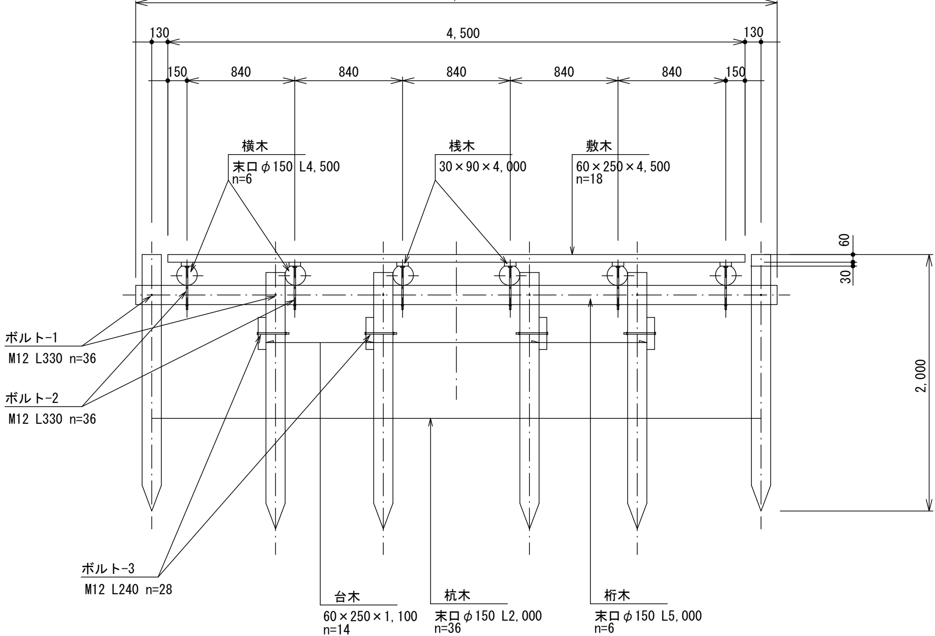
断面図 A--A
