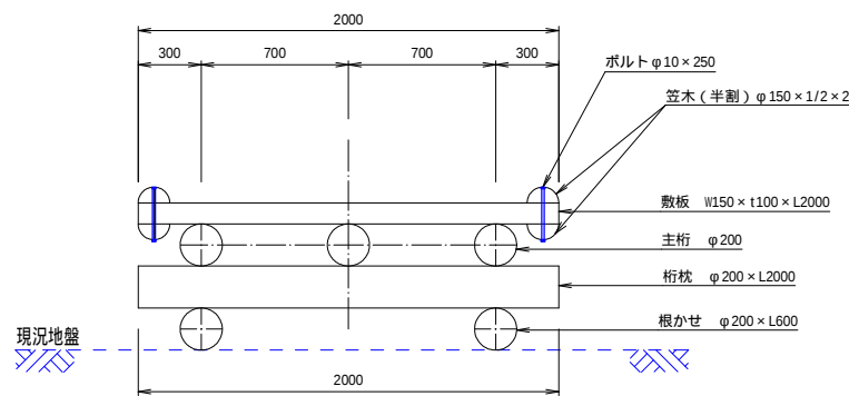
木道数量計算 (3.0m当り)
