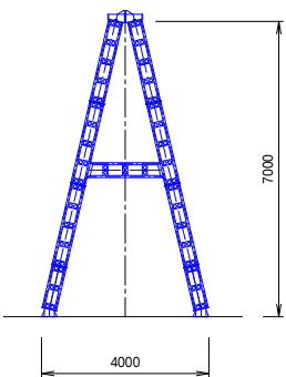
ケーブルクレーン索道用タワー A型柱：300×300×H7000
