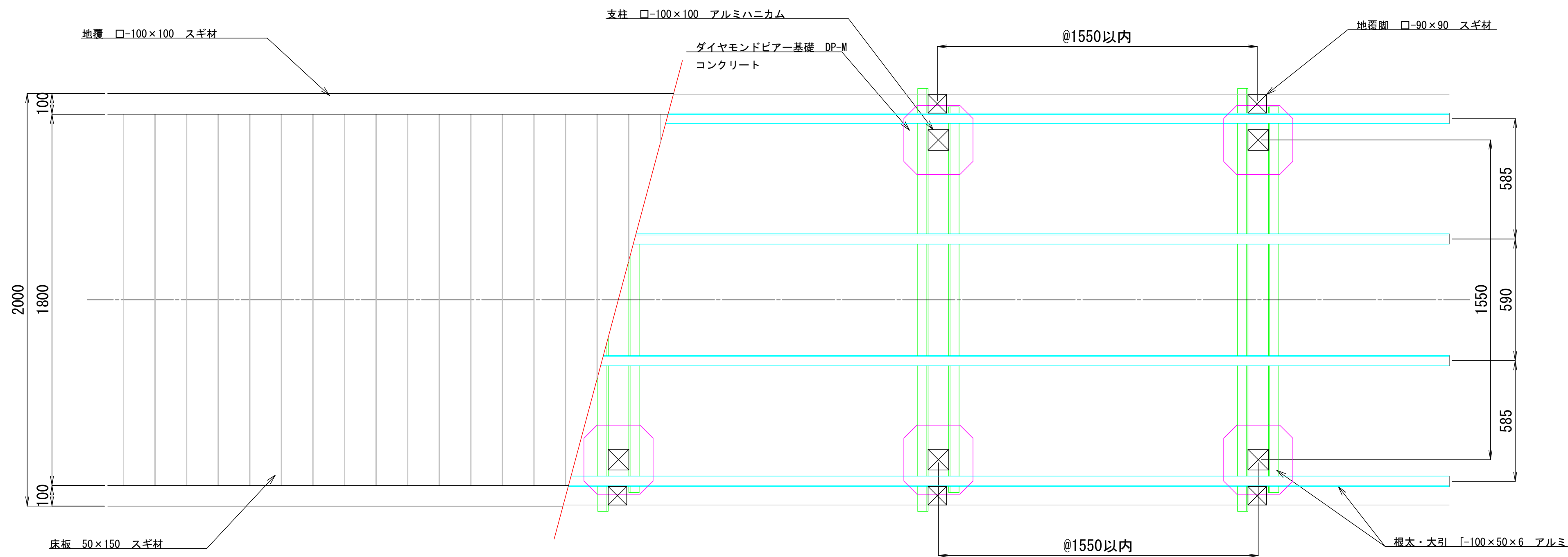
平面・根太伏図 S=1/15
