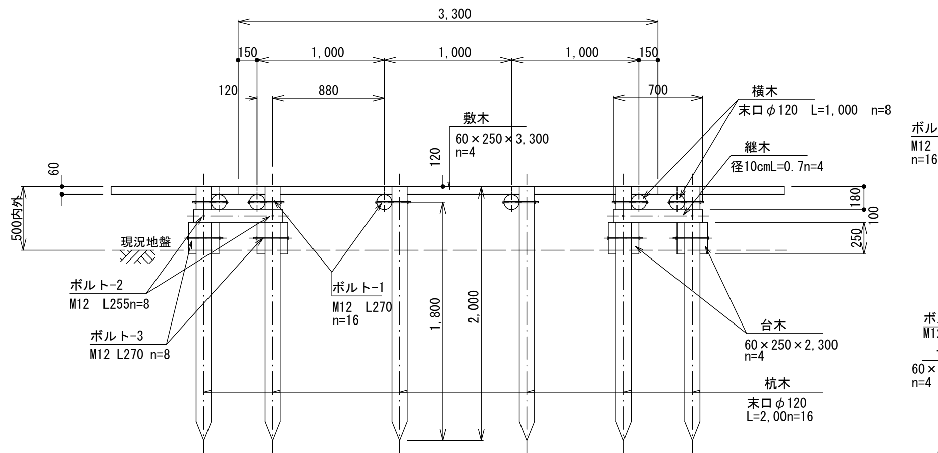
側面図
