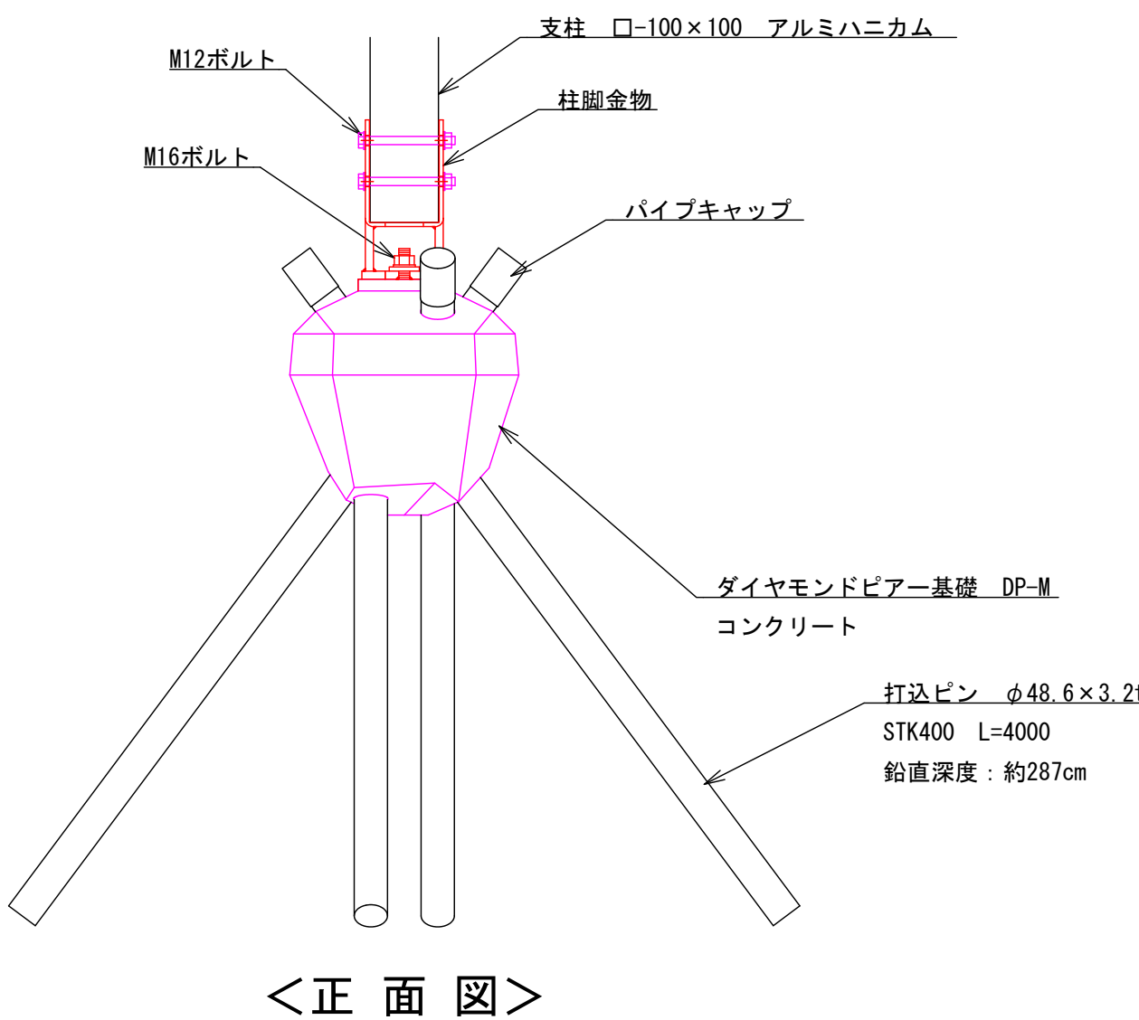
基礎詳細図 ～ダイヤモンドピア基礎 DP-M～
