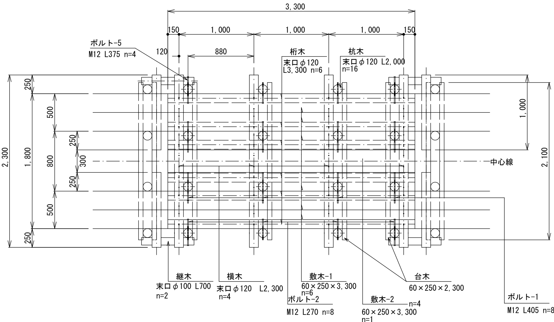
平面図
