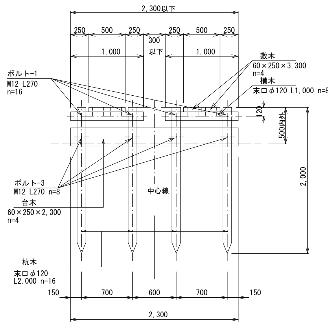
断面図
