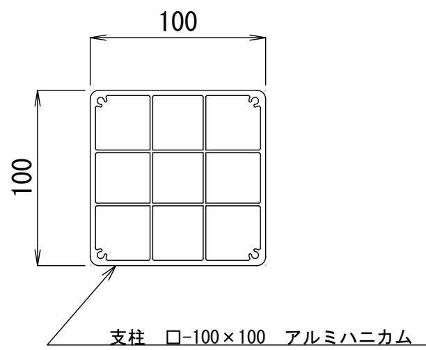
支柱断面図 S=1/3 (A1)、S=1/6 (A3)
