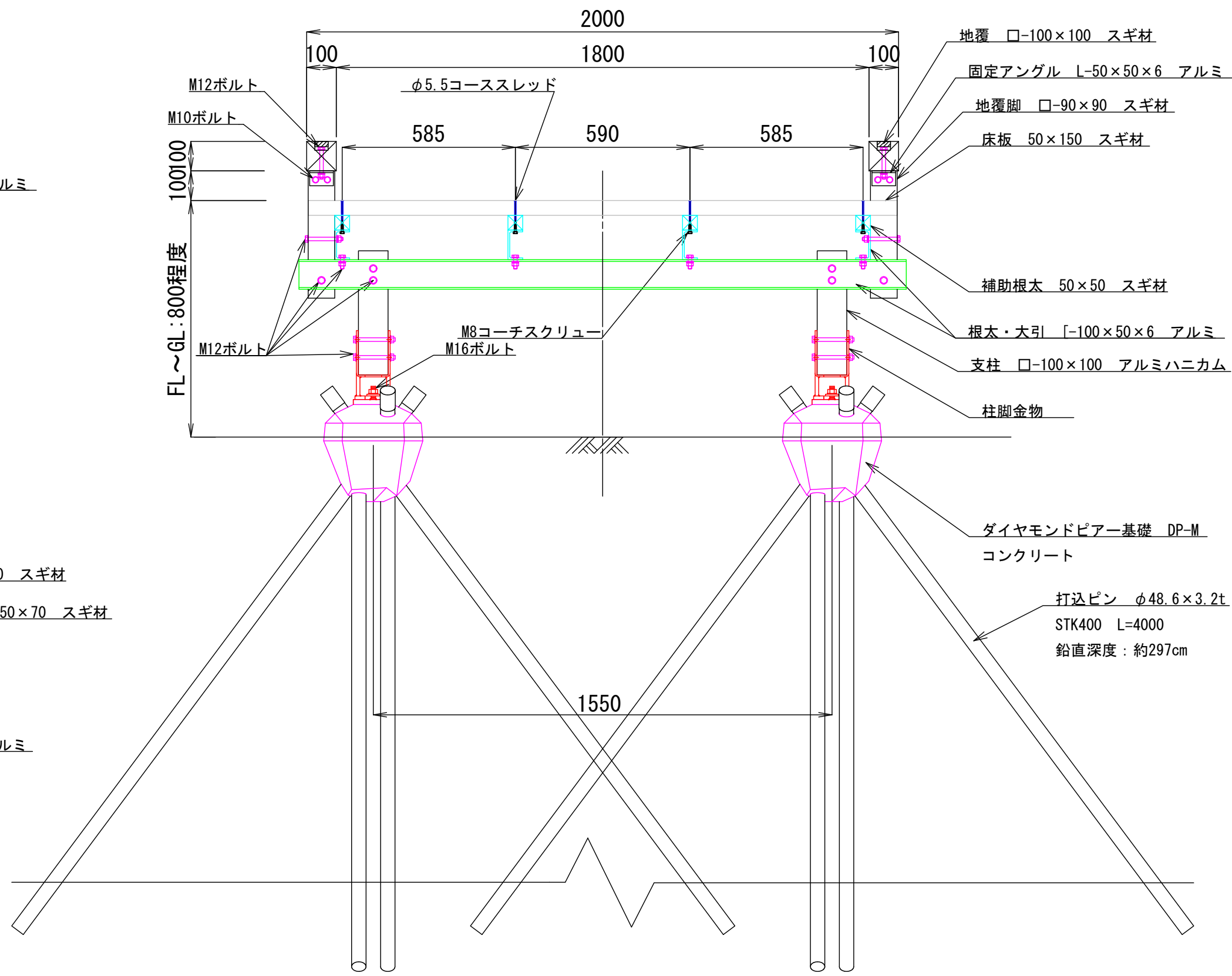
断面図 S=1/15
