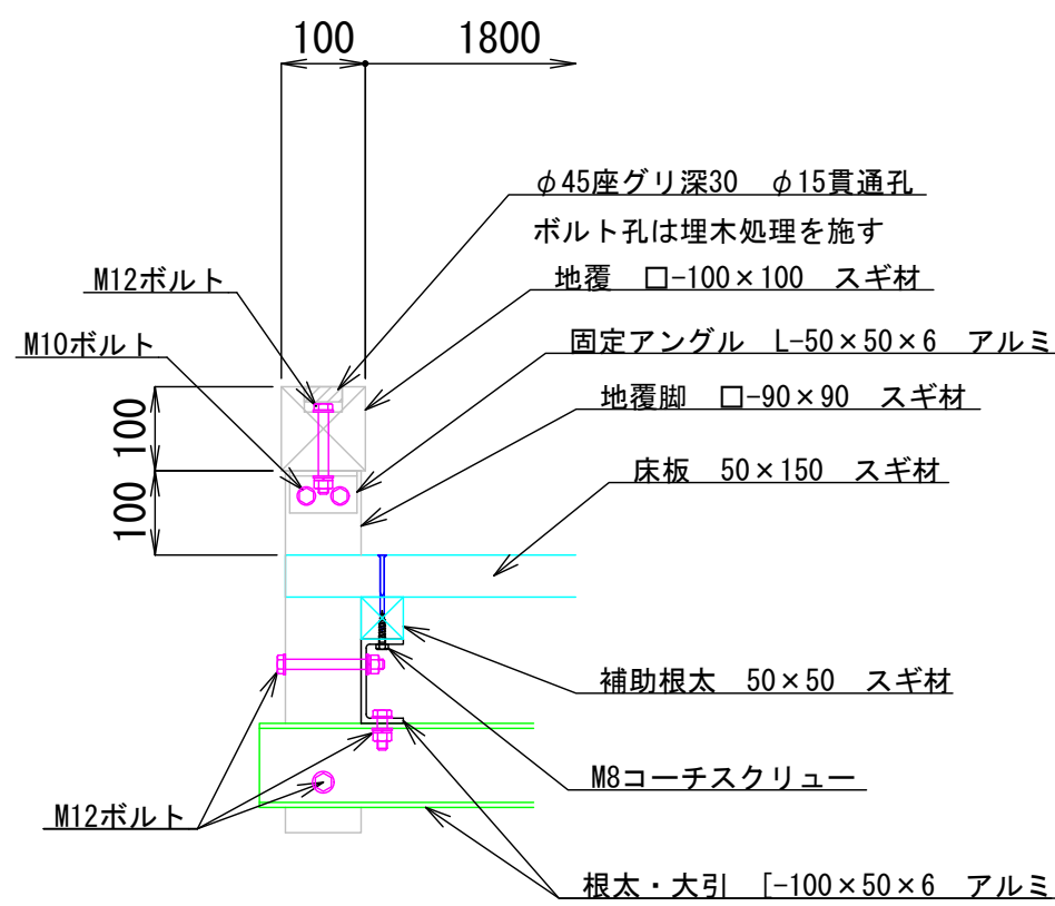
<断面図>
