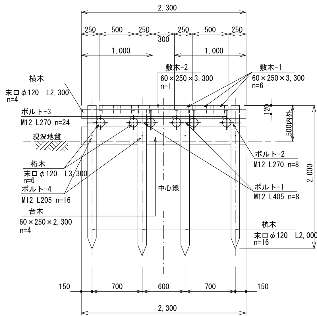
断面図
