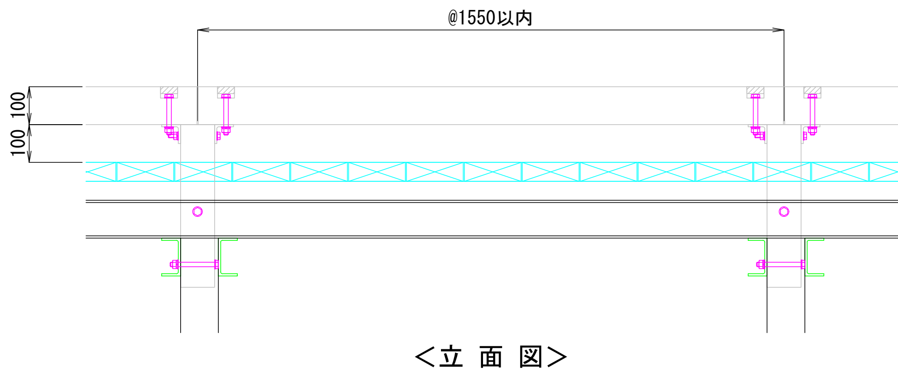
地覆詳細図
