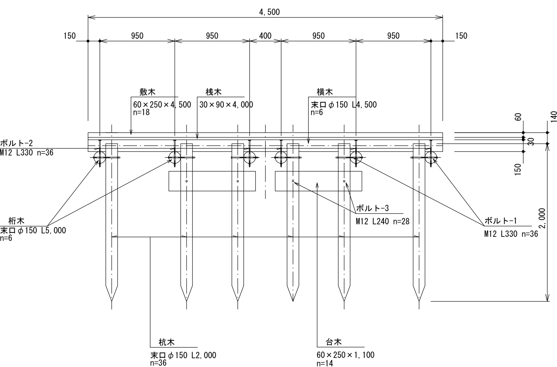
断面図 C--C
