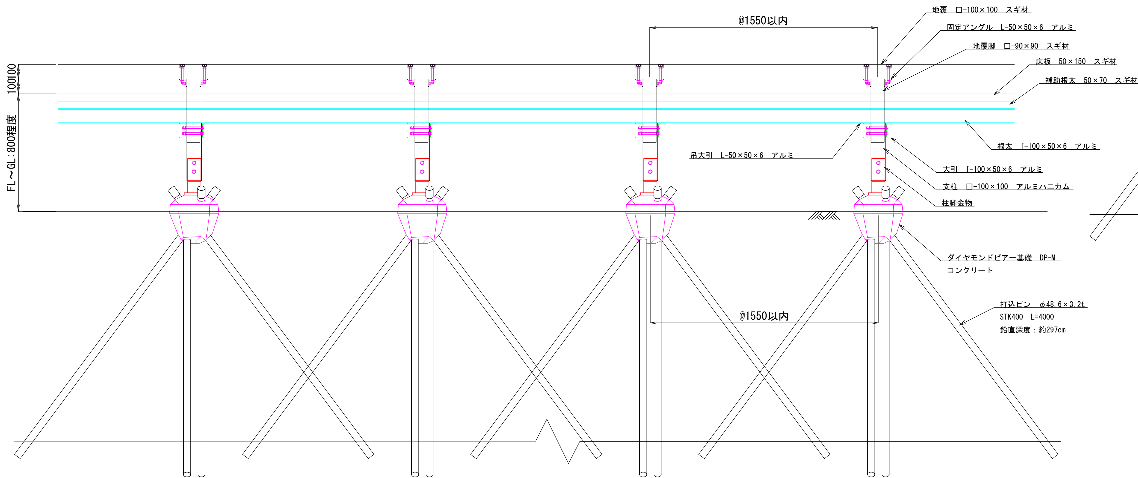
立面図 S=1/15
