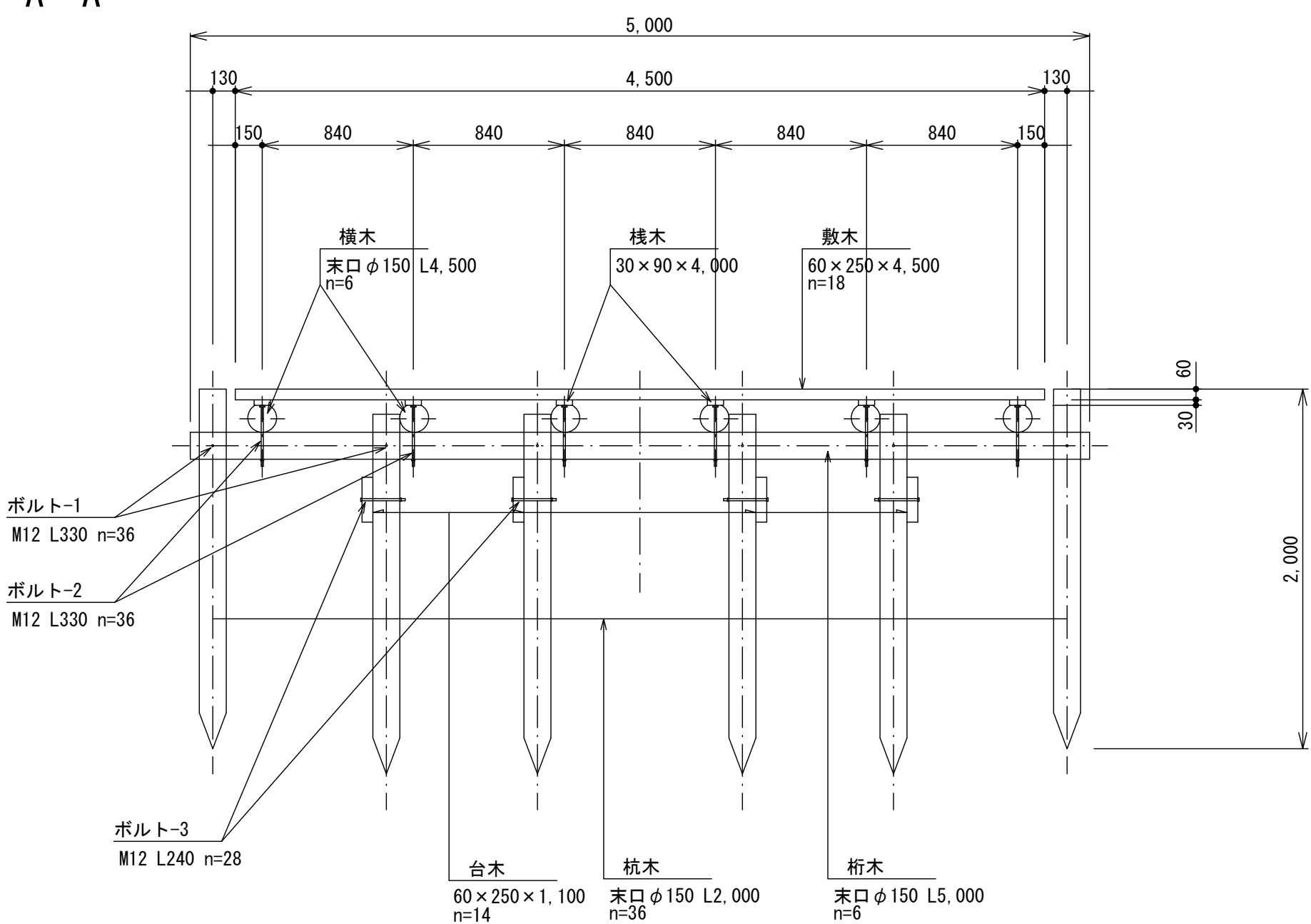
断面図 A--A
