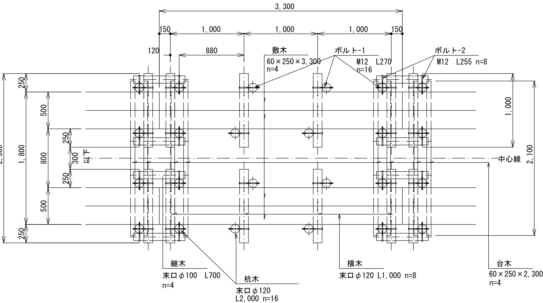
平面図
