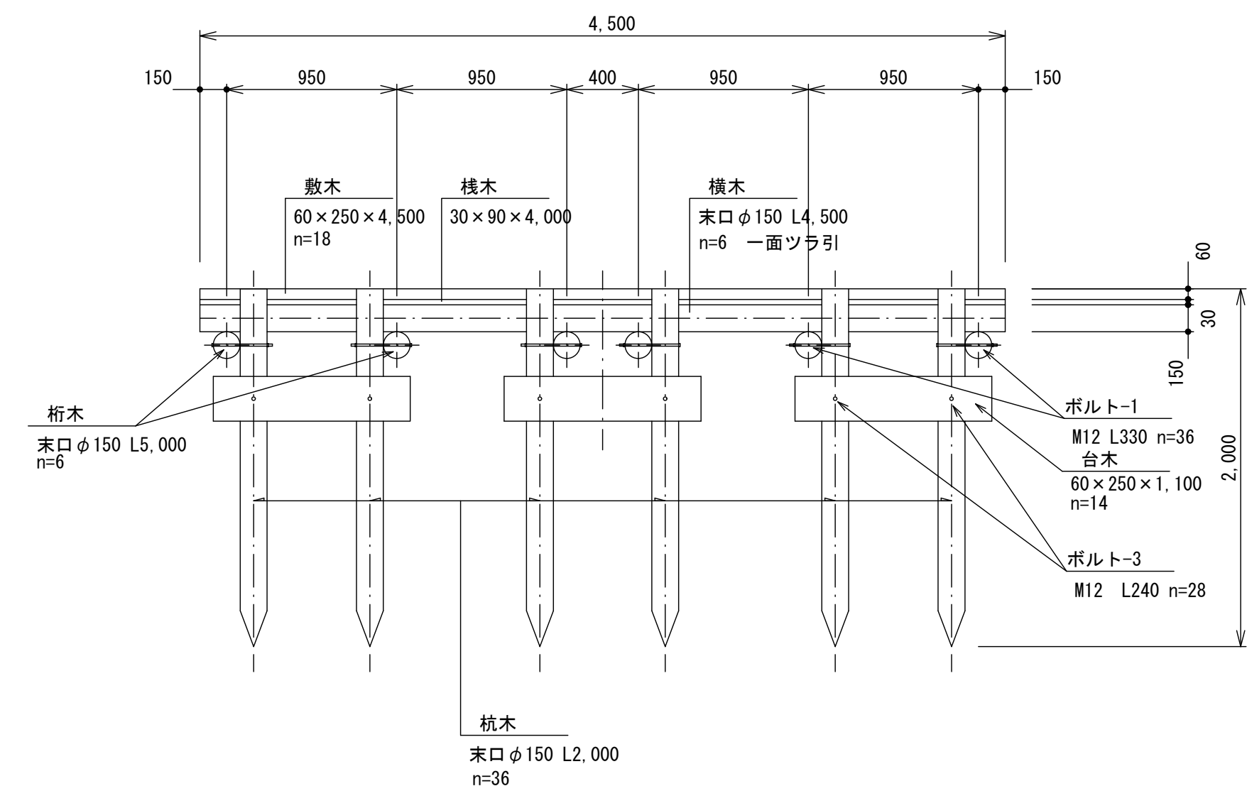
断面図 C--C
