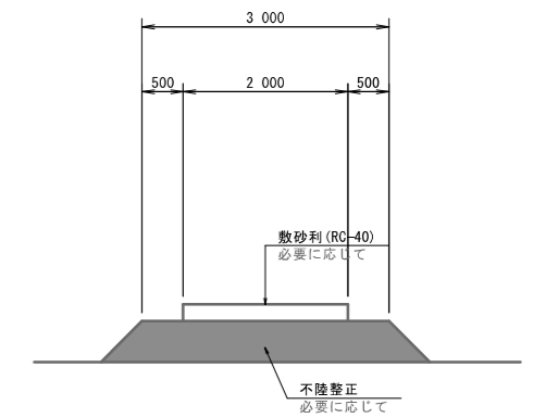
仮設道路参考図 S=1:50
