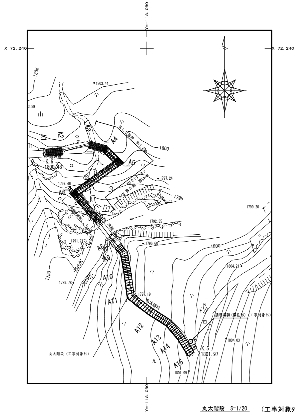
丸太階段 S=1/20 (工事対象外)
