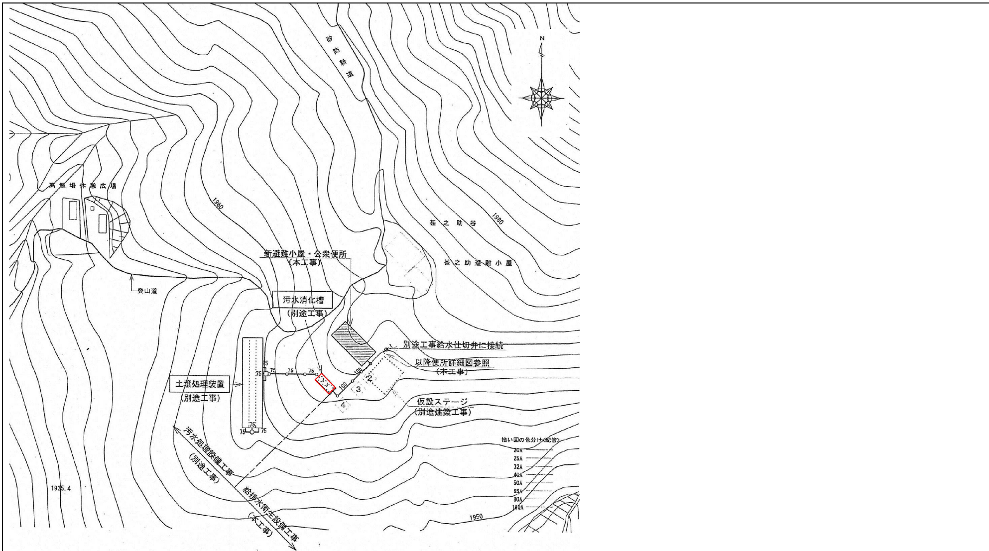
甚ノ助避難小屋配置図 1
