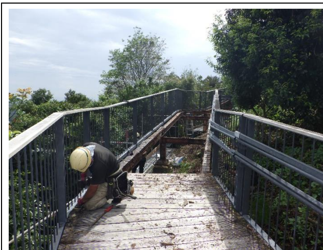
写真3 床板の撤去
