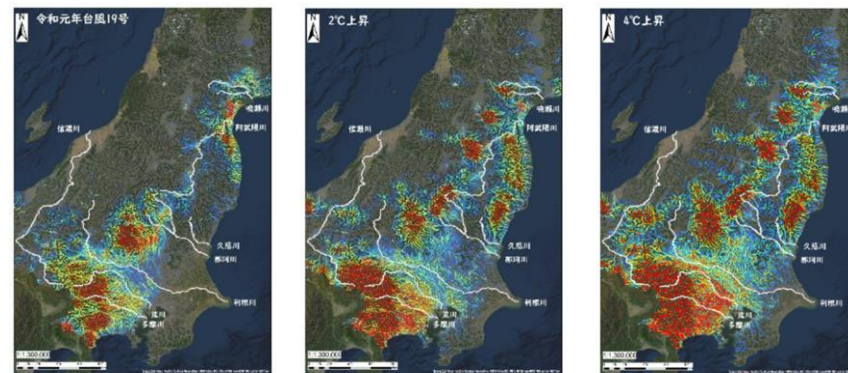
ピーク流出高の変化 (RRI, 2℃上昇, 4℃上昇シナリオは5ケースの平均を示す)
